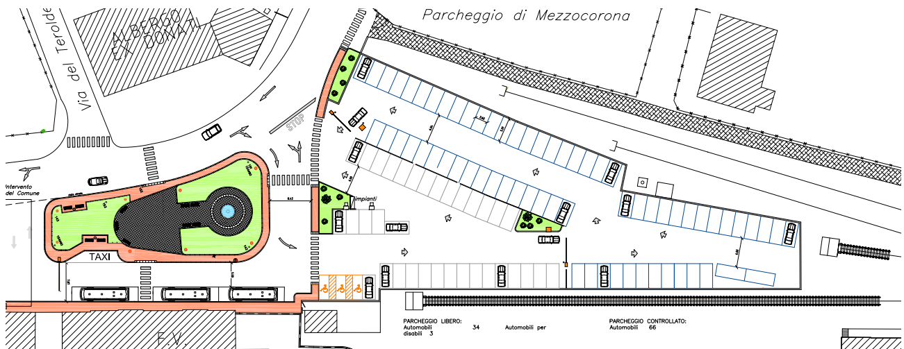
Progetto nuovi parcheggi in Piazza Trento
